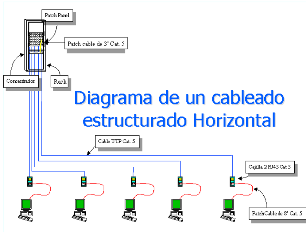
Figura 1.4: Subsistema Horizontal.
